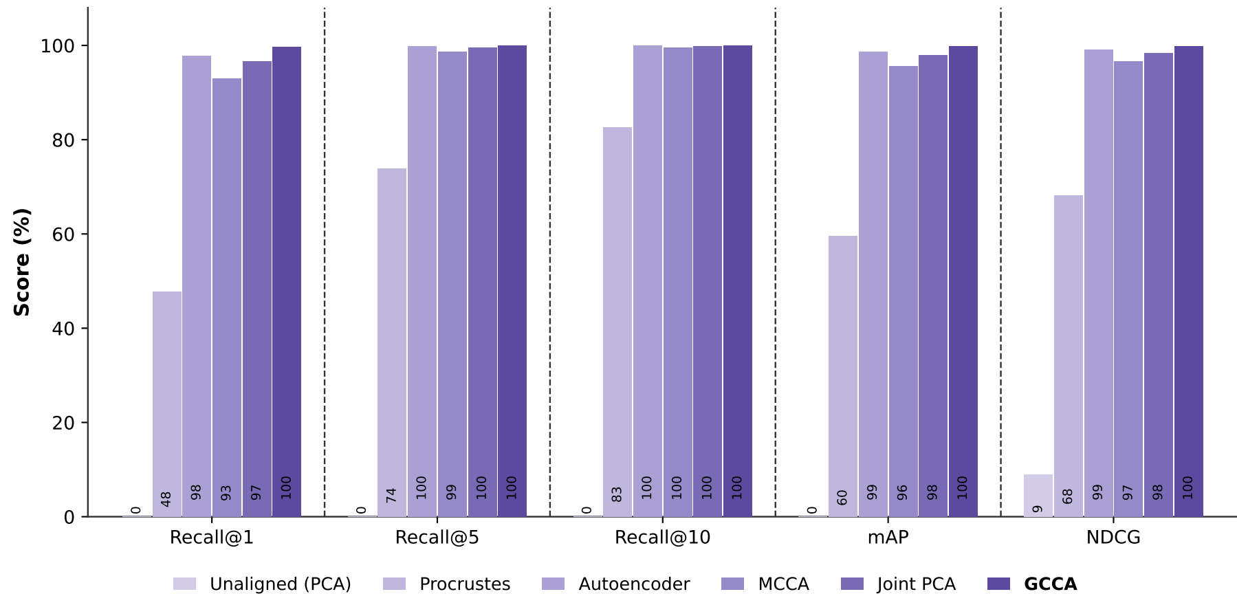
Cross-model retrieval — CPTAC · 5× · 224px
