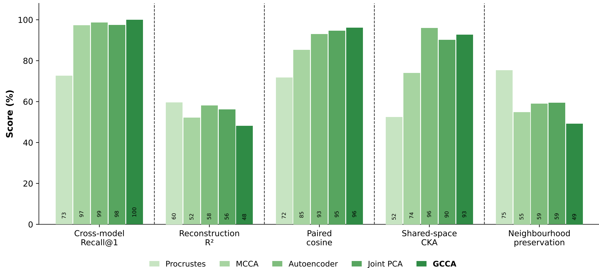
Alignment methods — TCGA · 10× · 224px
