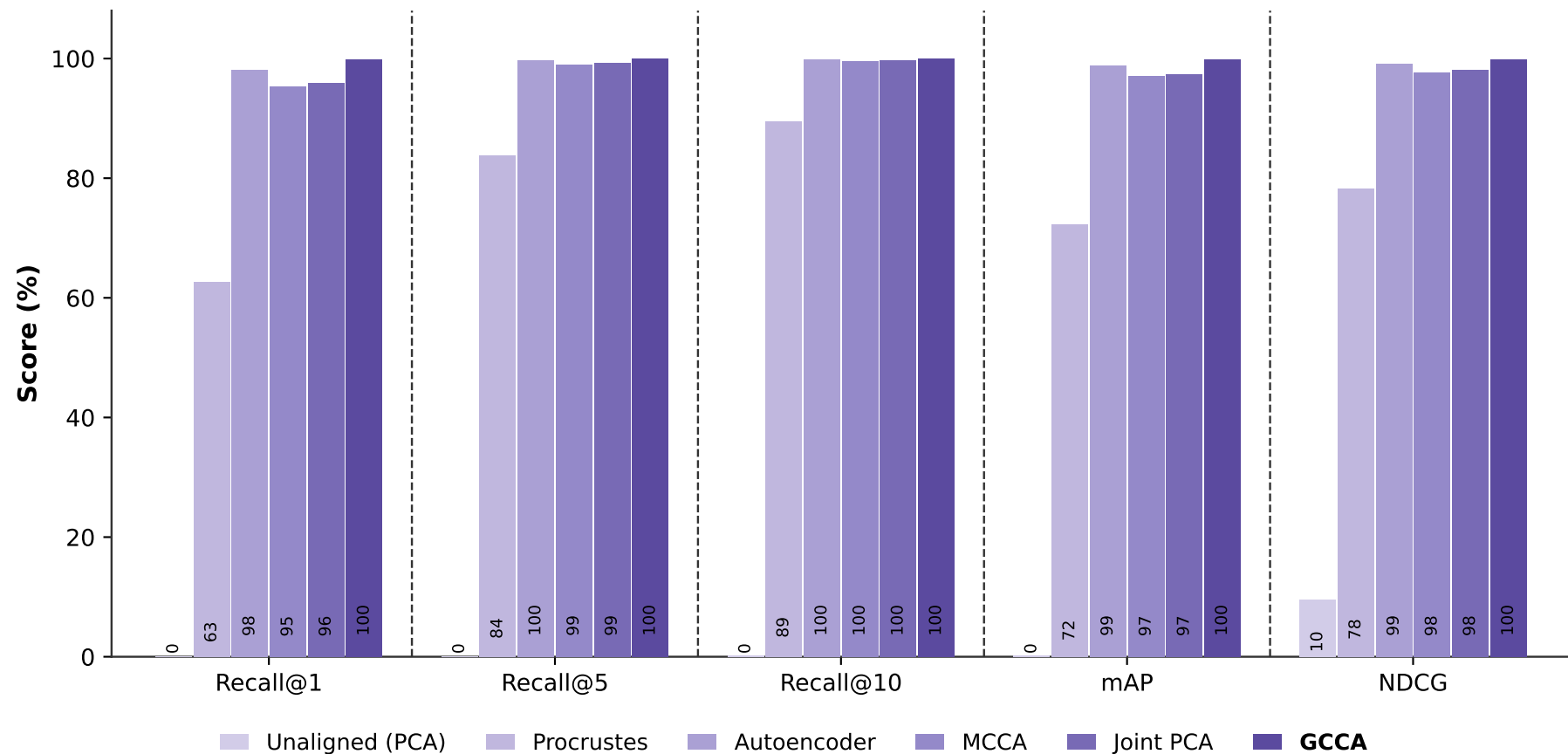
Cross-model retrieval — TCGA · 10× · 224px
