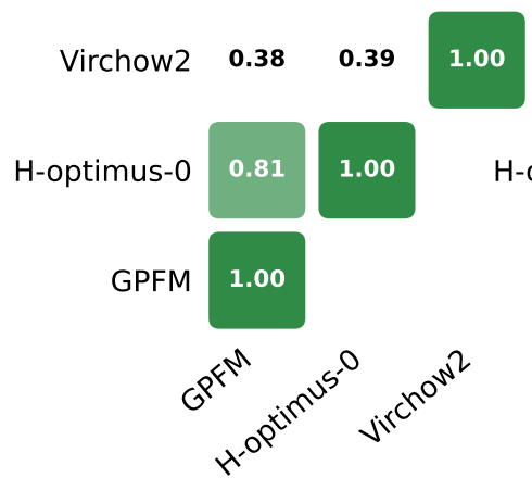
Linear CKA
