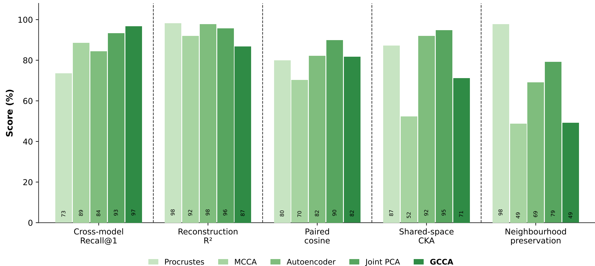
Alignment methods — TCGA · 10× · 512px (CONCH v1 / v1.5)
