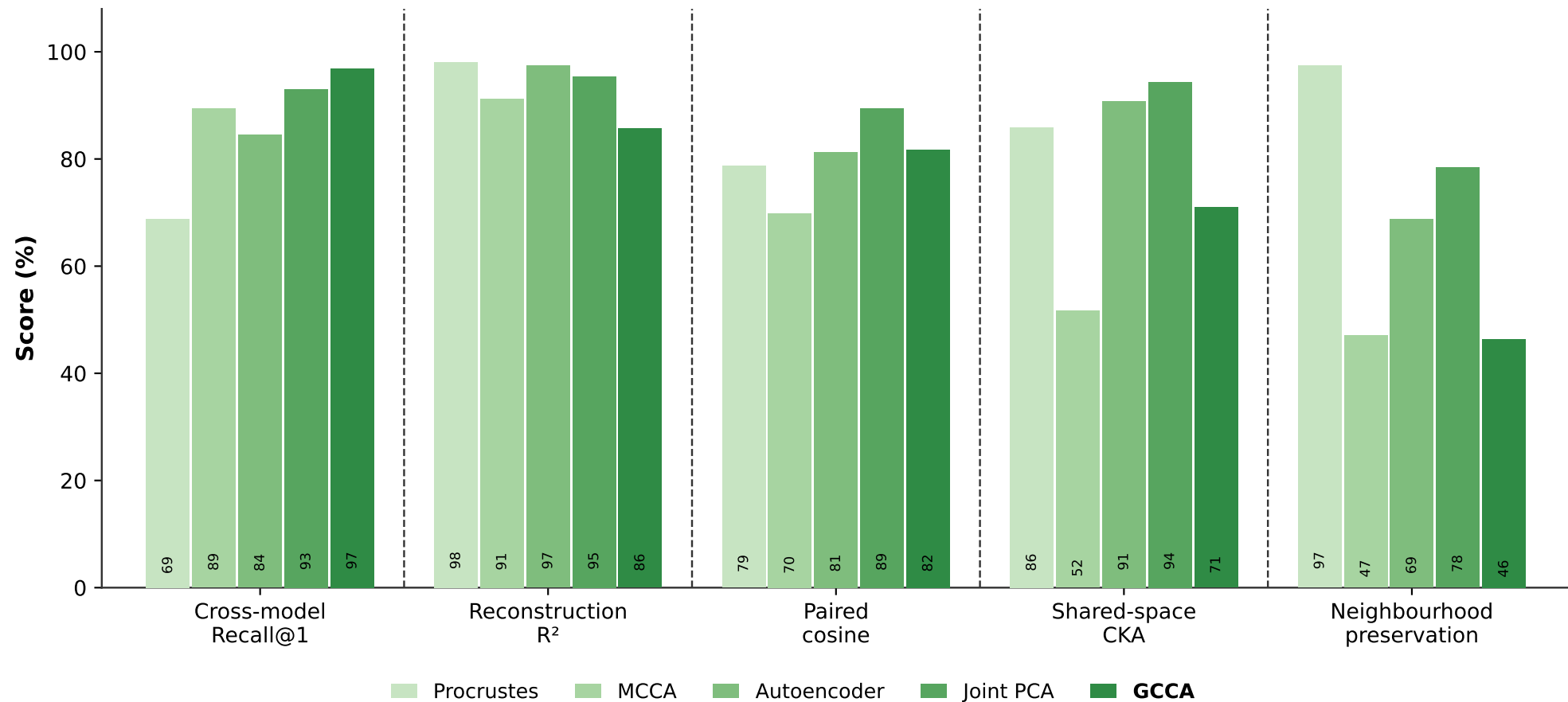
Alignment methods — TCGA · 20× · 512px (CONCH v1 / v1.5)
