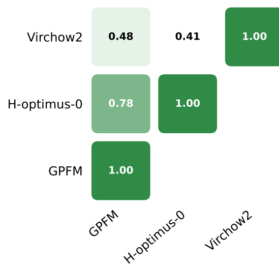
Linear CKA
