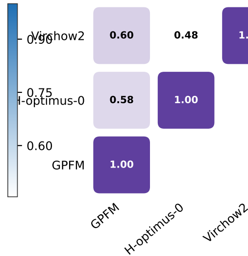
SVCCA
