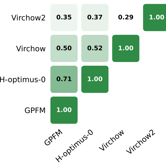
Linear CKA
