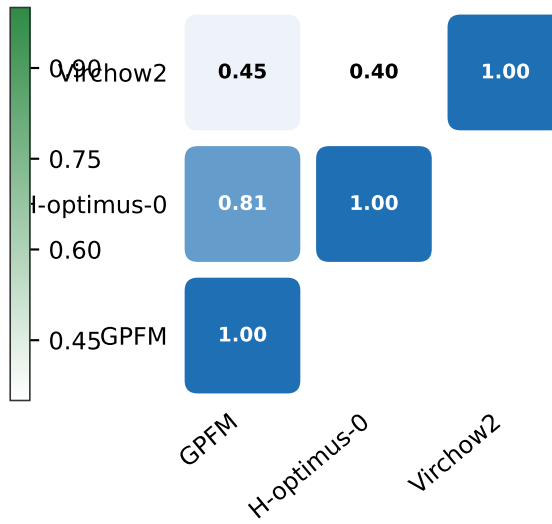
Kernel CKA
