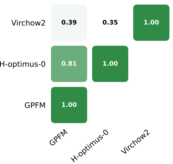
Linear CKA
