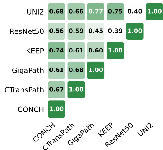
Linear CKA
