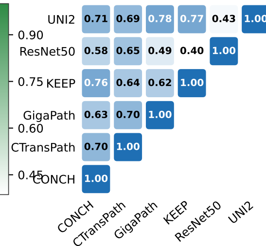
Kernel CKA
