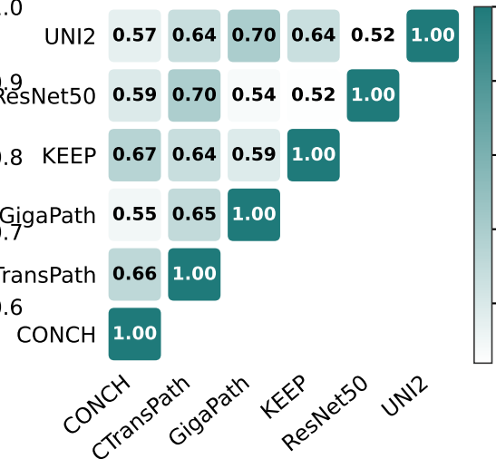
Procrustes
