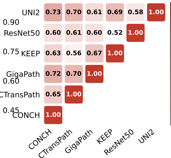
PWCCA
