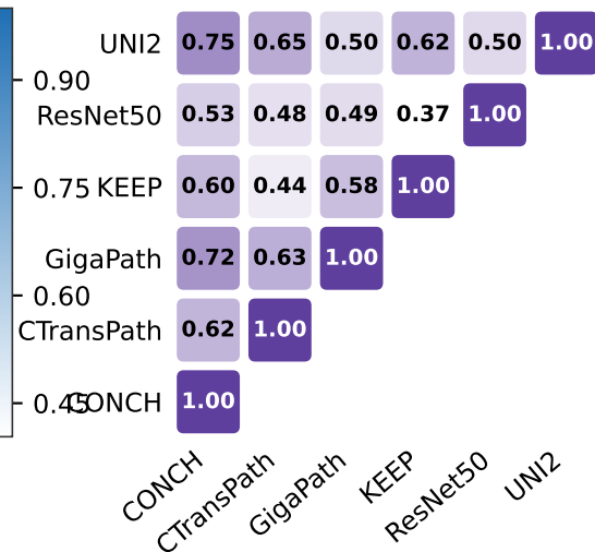
SVCCA
