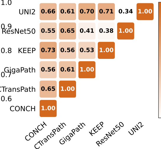
Cosine RSA
