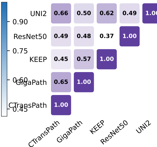
SVCCA
