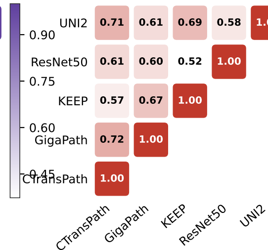
PWCCA
