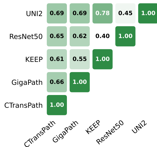
Linear CKA
