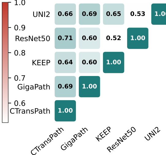
Procrustes
