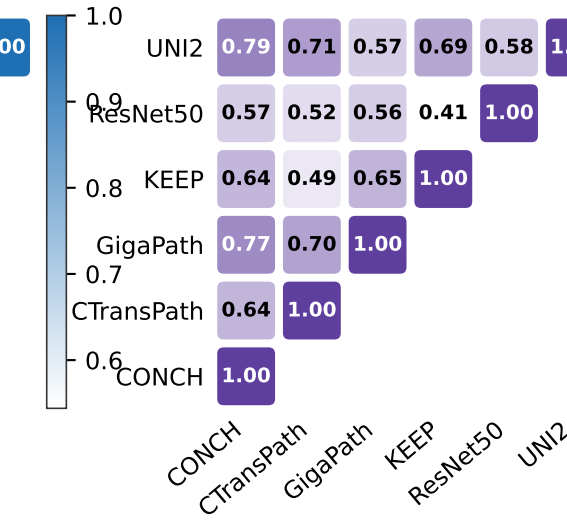
SVCCA
