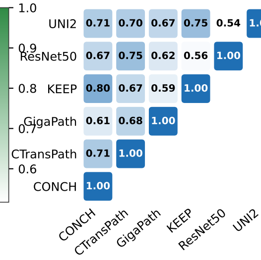
Kernel CKA
