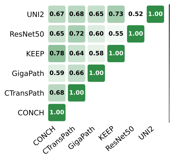
Linear CKA
