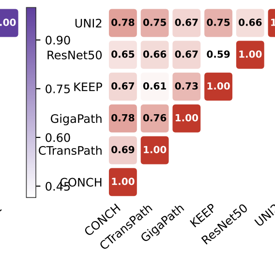
PWCCA
