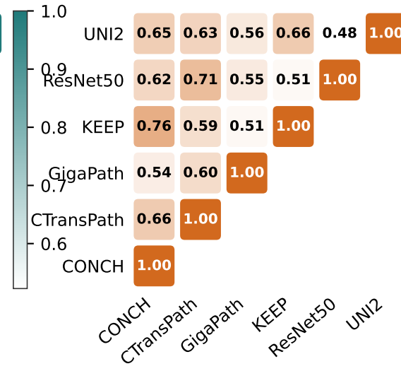
Cosine RSA
