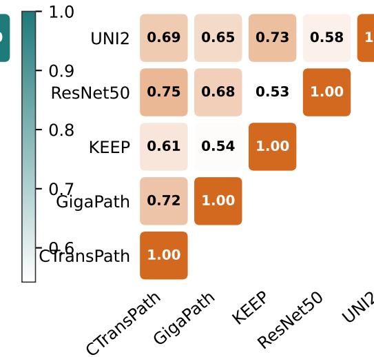
Cosine RSA
