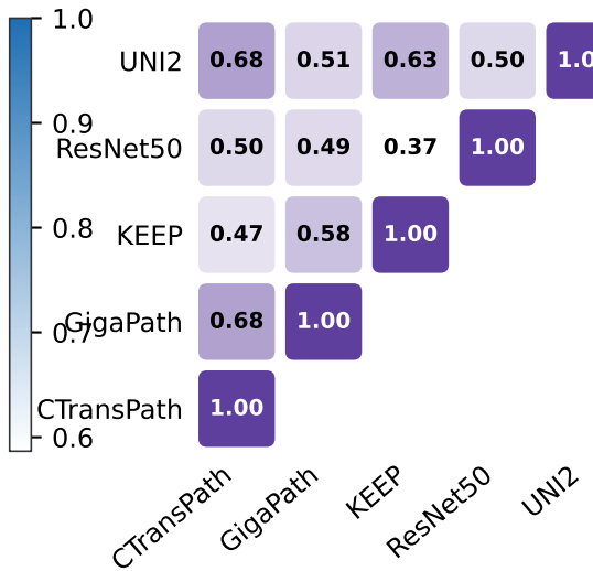
SVCCA
