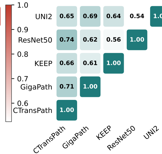
Procrustes
