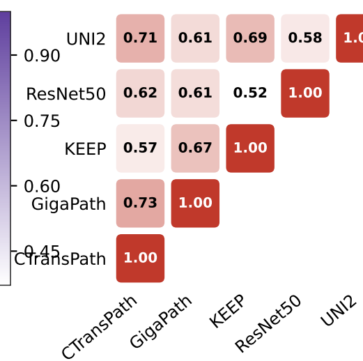
PWCCA
