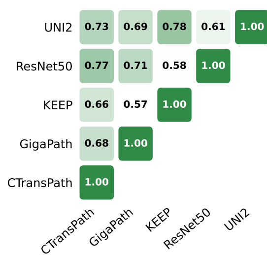
Linear CKA
