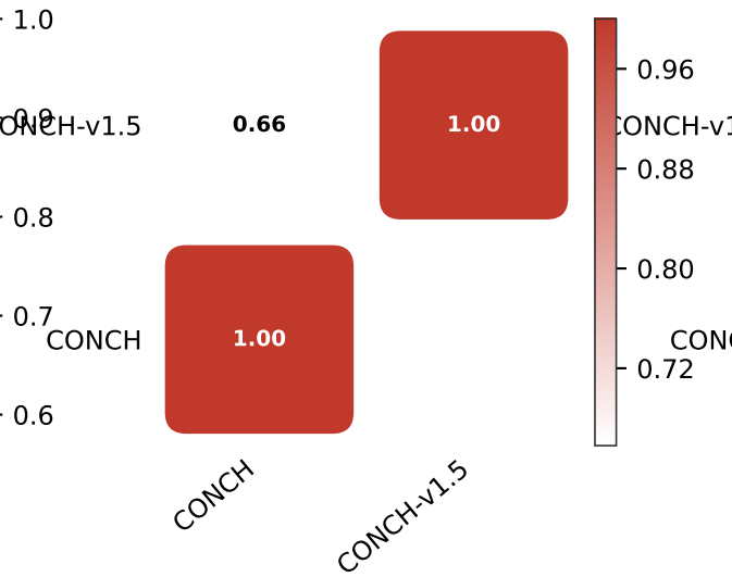
PWCCA
