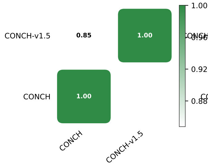
Linear CKA
