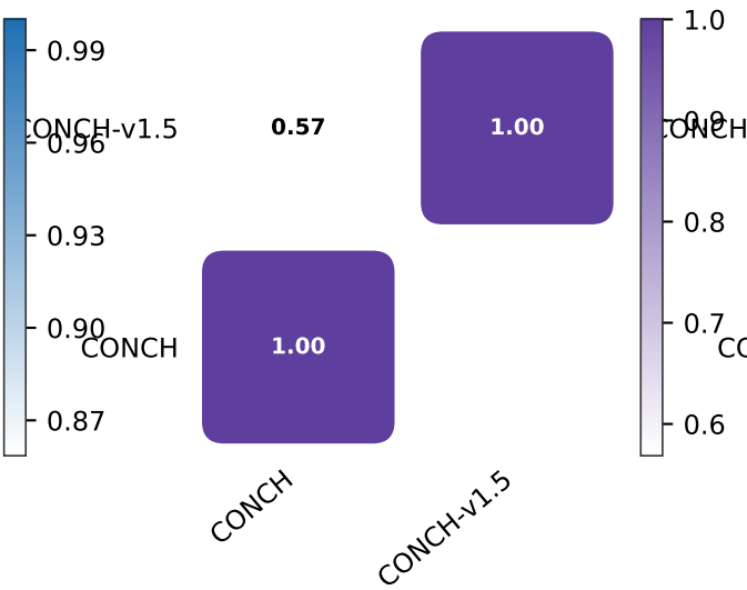
SVCCA
