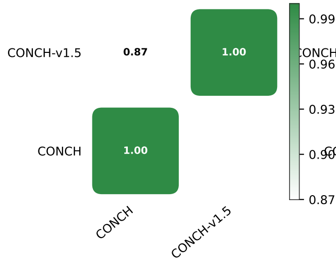
Linear CKA
