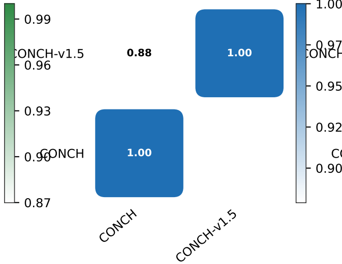
Kernel CKA
