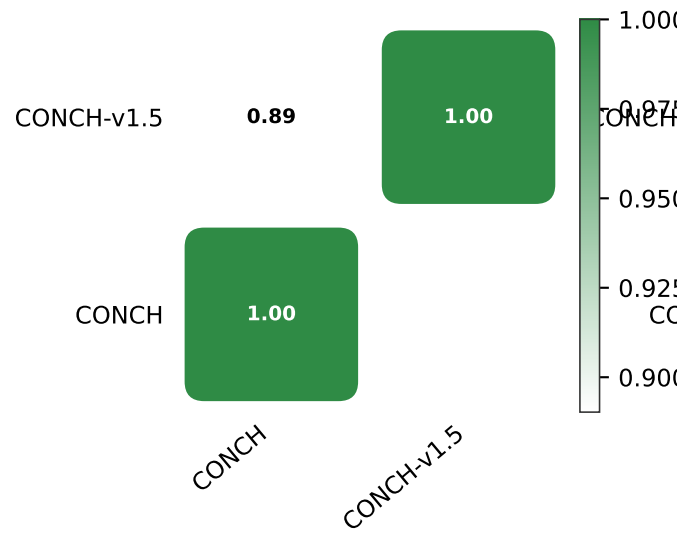
Linear CKA
