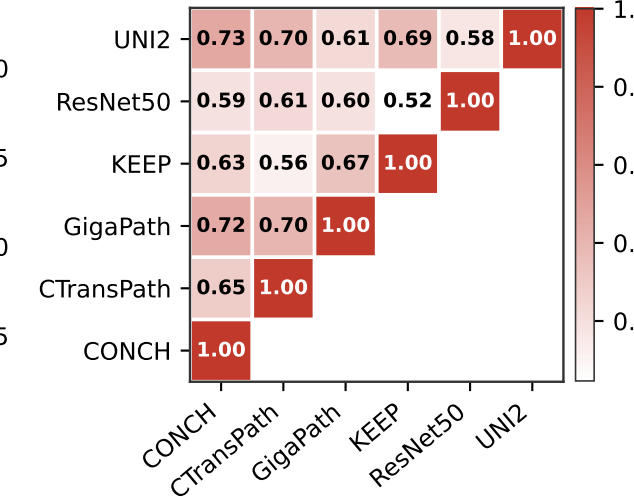
PWCCA
