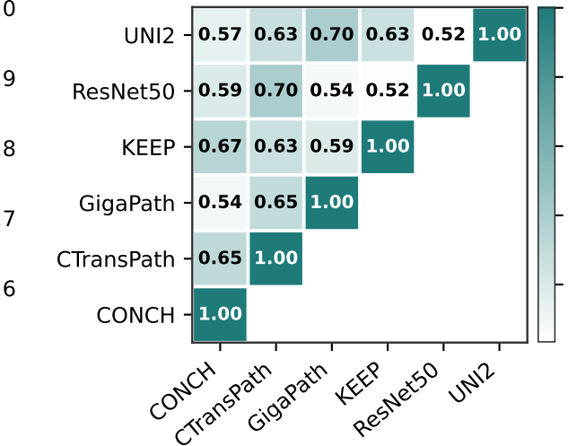
Procrustes
