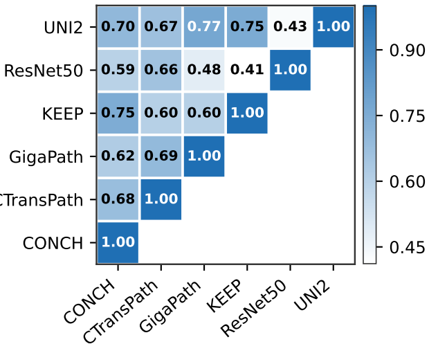
Kernel CKA
