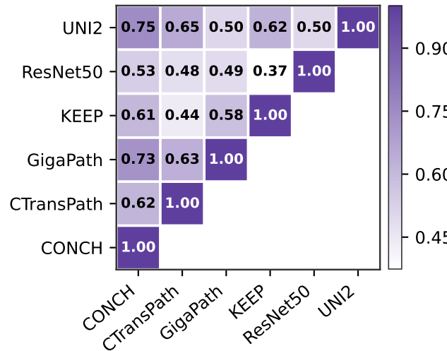
SVCCA
