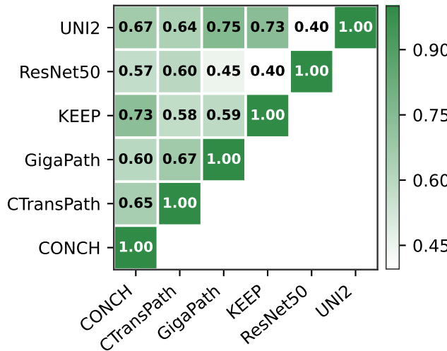
Linear CKA
