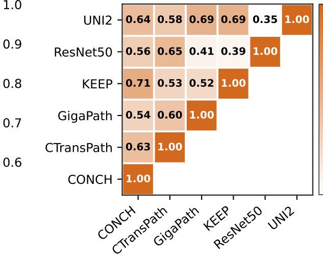
Cosine RSA
