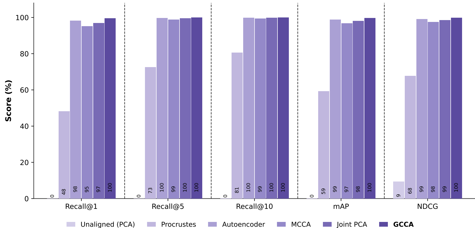
Cross-model retrieval — CPTAC · 20× · 224px (Virchow / GPFM / H-optimus)
