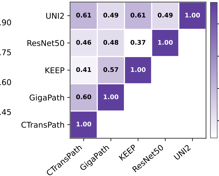
SVCCA
