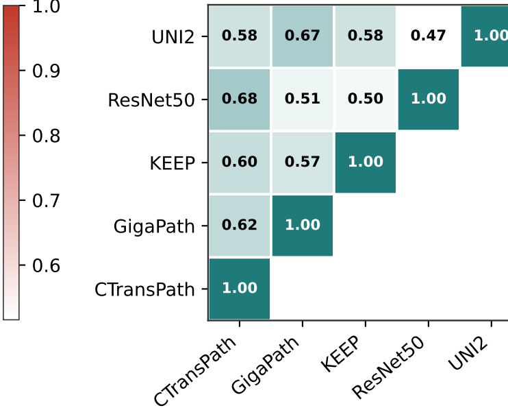
Procrustes
