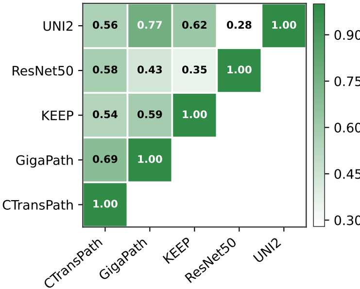
Linear CKA
