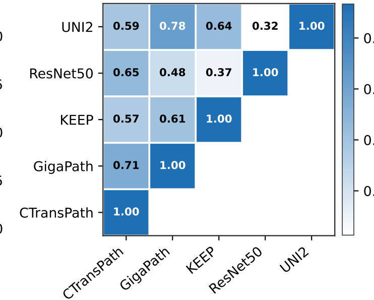
Kernel CKA
