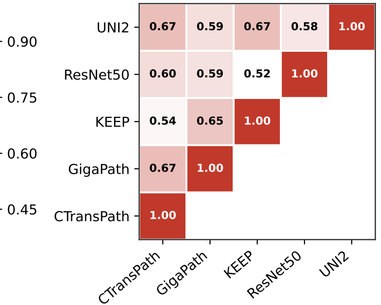
PWCCA
