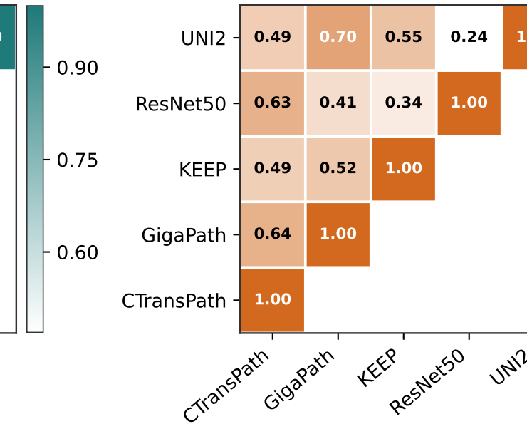
Cosine RSA
