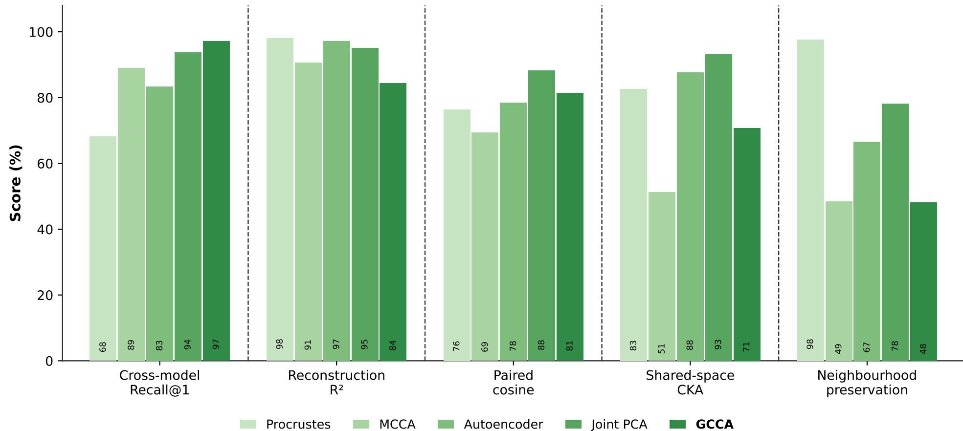
Alignment methods — CPTAC · 20× · 512px (CONCH v1 / v1.5)
