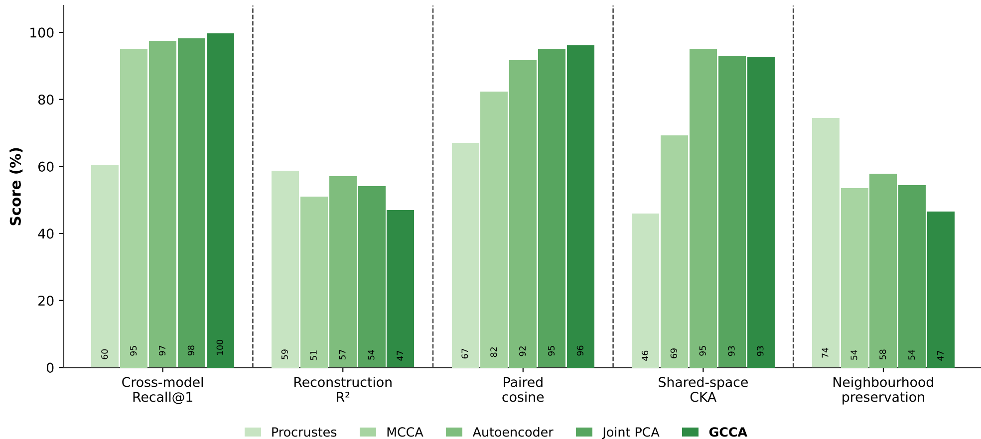
Alignment methods — TCGA · 20× · 224px (Virchow / GPFM / H-optimus)
