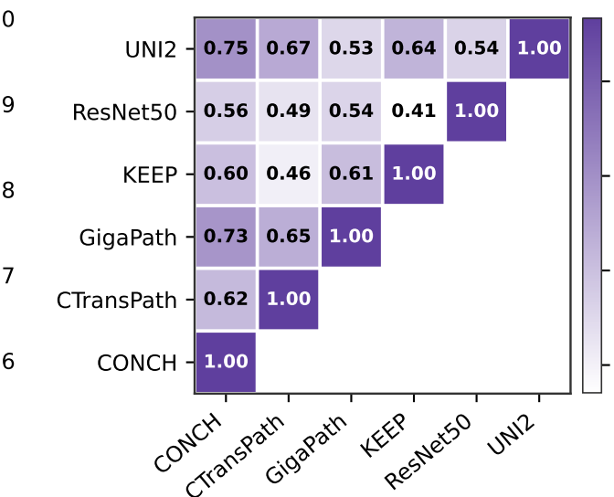
SVCCA
