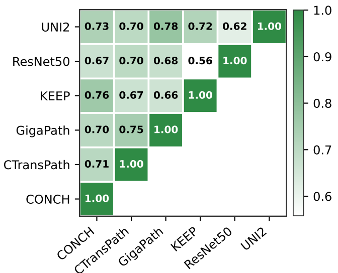
Linear CKA
