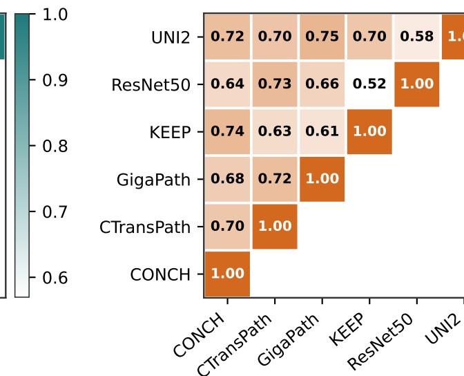
Cosine RSA
