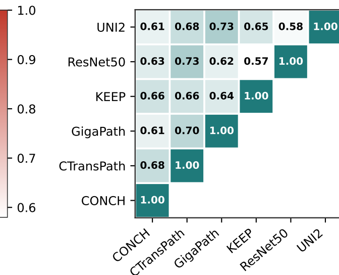
Procrustes
