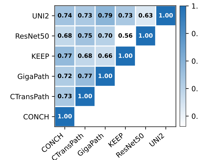
Kernel CKA
