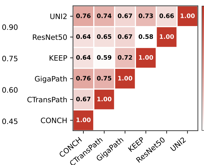
PWCCA
