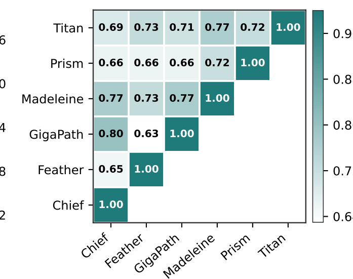
Procrustes
