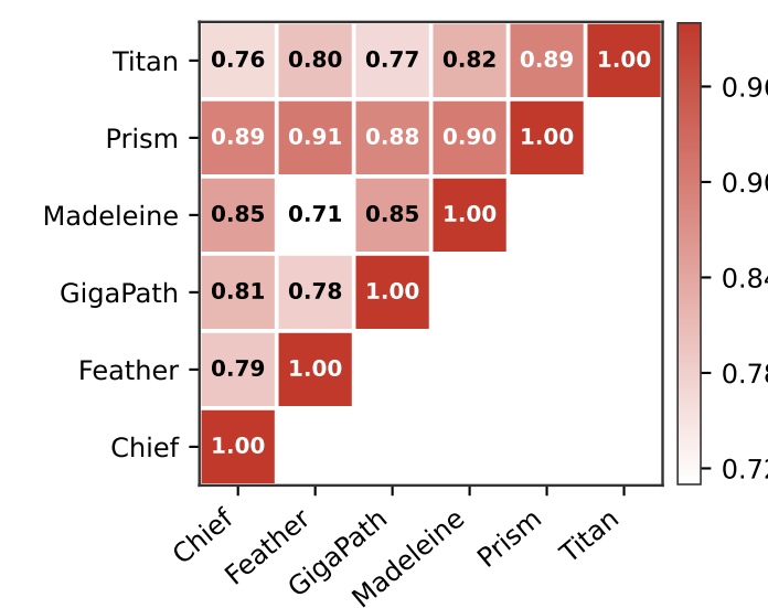
PWCCA
