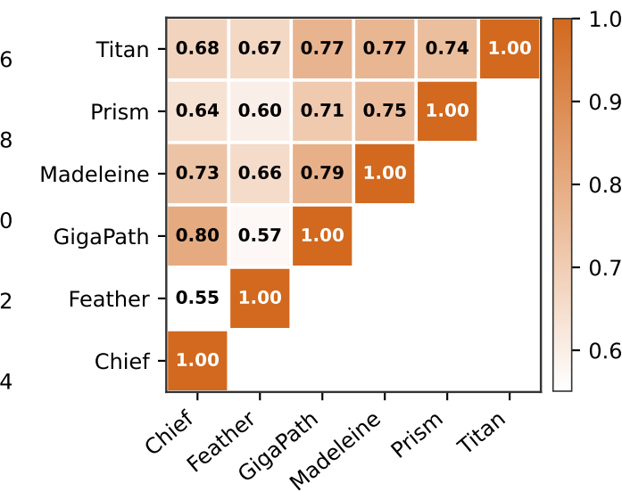
Cosine RSA
