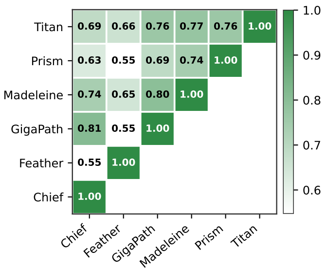
Linear CKA
