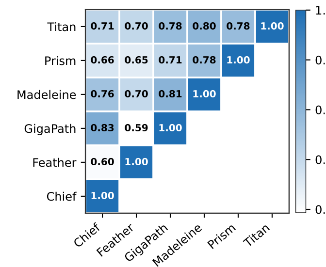
Kernel CKA
