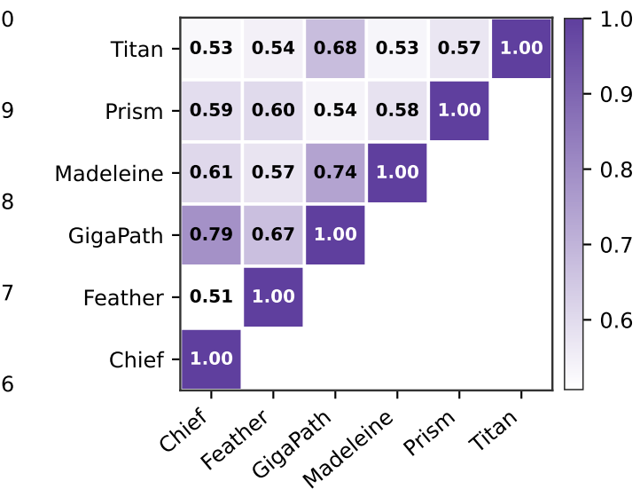
SVCCA
