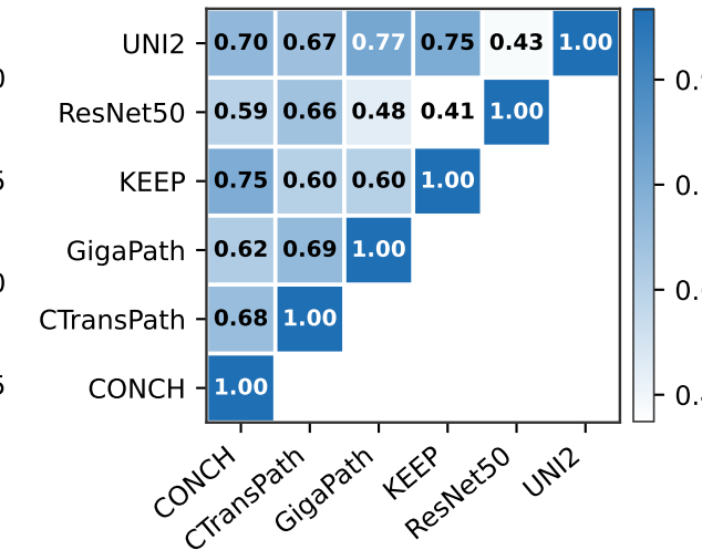
Kernel CKA
