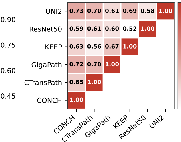
PWCCA
