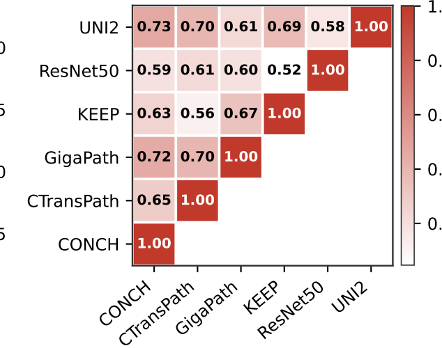
PWCCA
