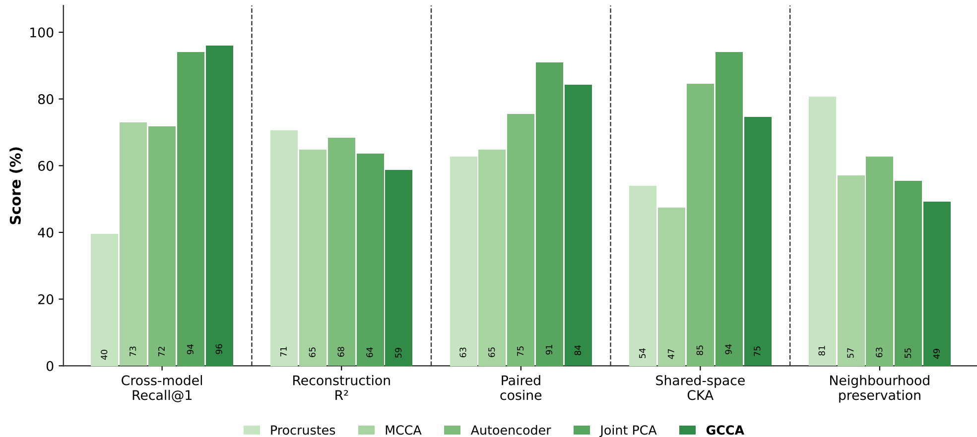
Alignment methods — CPTAC · 20× · 256px
