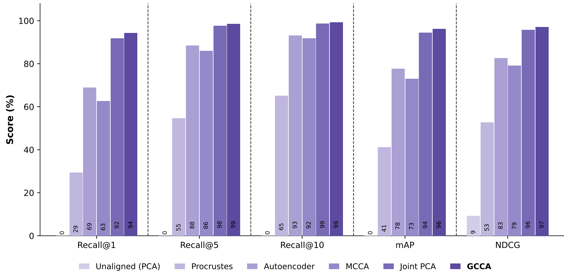
Cross-model retrieval — CPTAC · 20× · 256px
