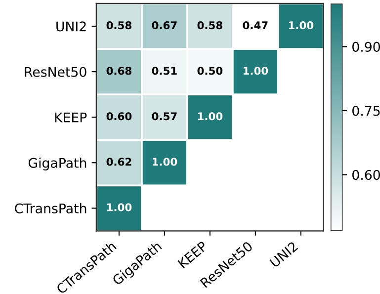
Procrustes
