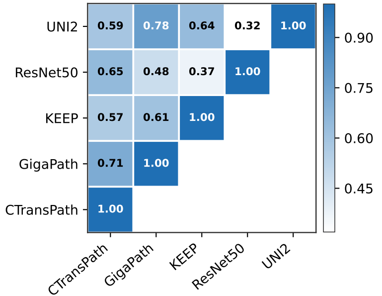
Kernel CKA
