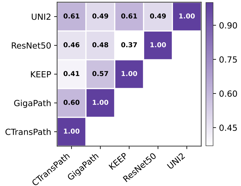
SVCCA
