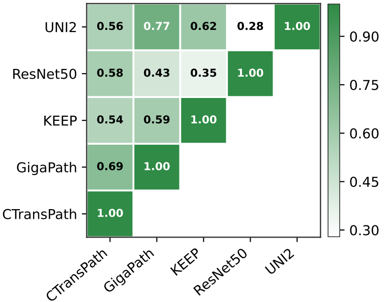
Linear CKA
