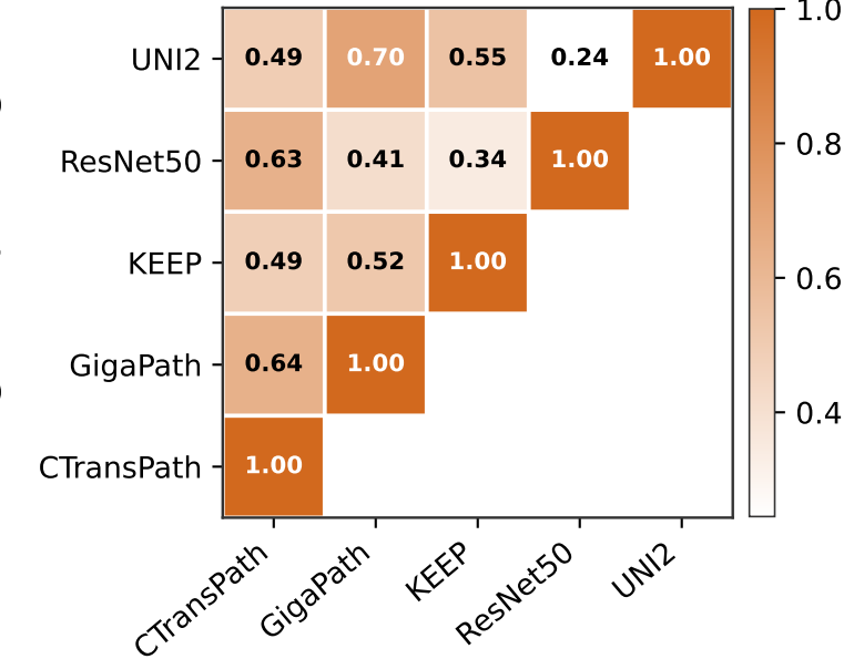
Cosine RSA
