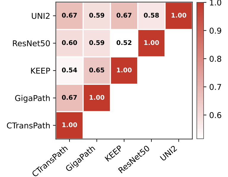
PWCCA
