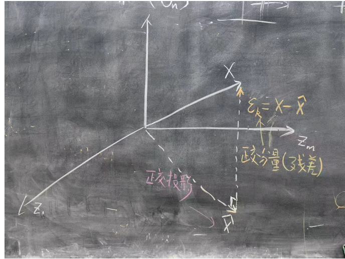
图 1: 正交投影的几何表示。
