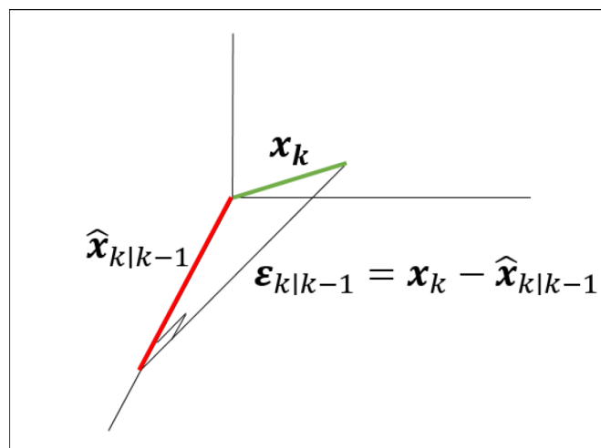
图 2: 先验估计 \hat{\mathbf{x}}_{k|k-1} 及其误差 \boldsymbol{\varepsilon}_{k|k-1}
