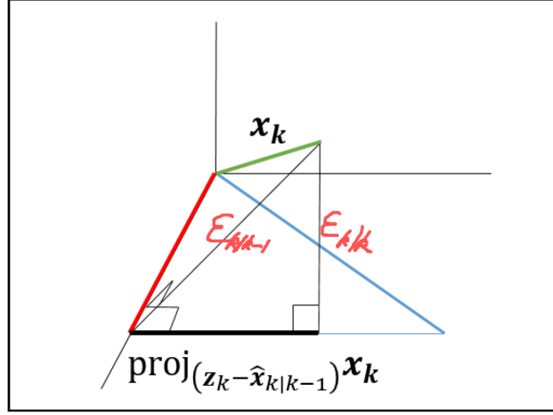
图 4: 真实状态 \mathbf{x}_k 投影到新息 \tilde{\mathbf{z}}_k 上
