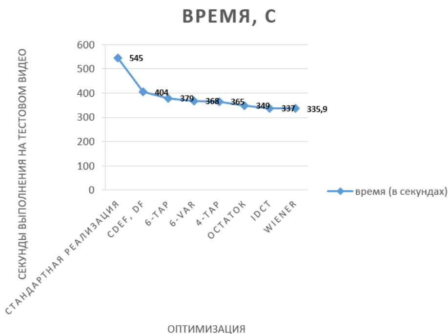
Рис. 31 – зависимость времени декодирования от оптимизаций
