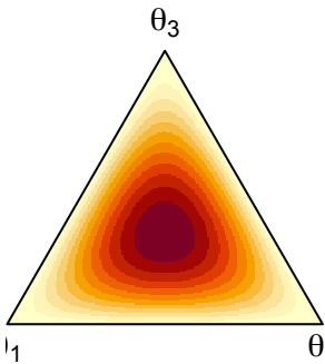
Dirichlet(2,2,2)
