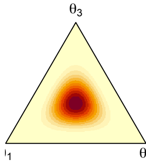
Dirichlet(5,5,5)
