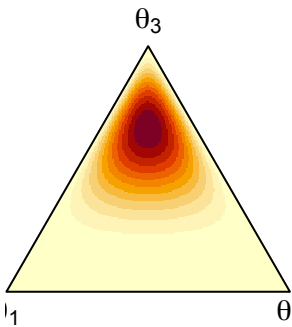
Dirichlet(2,2,5)
