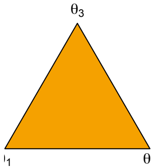
Dirichlet(1,1,1)
