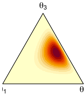
Dirichlet(2,5,5)
