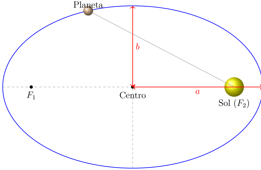
Figura 3.20: Ilustración de la Primera Ley de Kepler. La órbita del planeta es una elipse, con el Sol situado en uno de sus dos focos ( F_2 ). Se muestran el semieje mayor ( a ) y el semieje menor ( b ).
