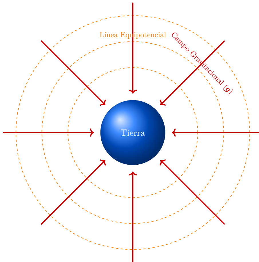
Figura 3.12: Representación en 2D del campo gravitacional ( g ) generado por la Tierra. Las líneas de campo (flechas rojas) son radiales y apuntan hacia el centro de masa. Las líneas equipotenciales (círculos naranjas a trazos) son perpendiculares a las líneas de campo.
