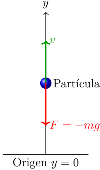
Figura 3.4: Diagrama de cuerpo libre para una partícula en lanzamiento vertical hacia arriba. El origen de coordenadas se sitúa en el punto de lanzamiento. Se muestra el vector velocidad ( v ) apuntando hacia arriba y el vector de la fuerza gravitacional ( F ) apuntando hacia abajo.
