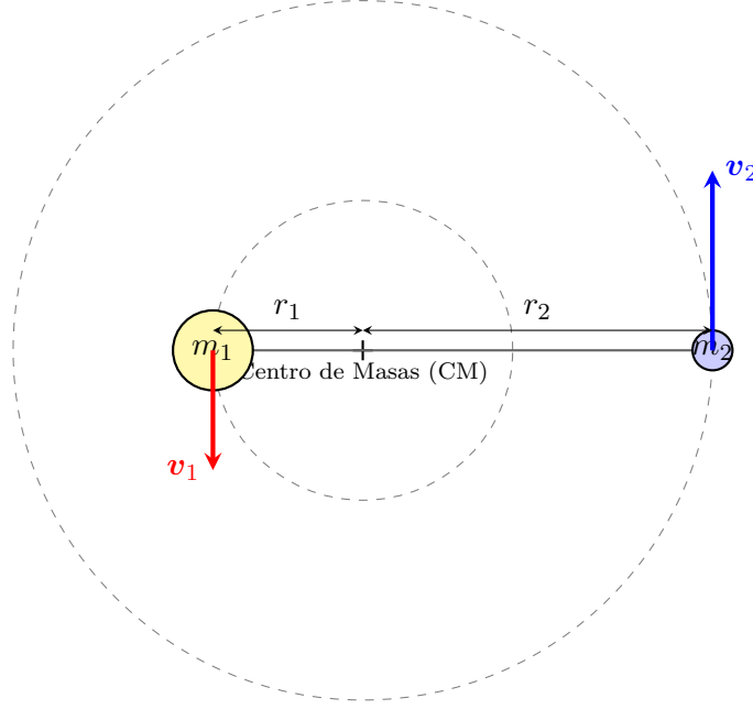
Figura 3.6: Un sistema binario orbitando su centro de masas común. Las cantidades de movimiento de ambos cuerpos ( \mathbf{p}_1 y \mathbf{p}_2 ) son siempre iguales en magnitud y opuestas en dirección, garantizando que el momento total sea cero respecto al CM.
