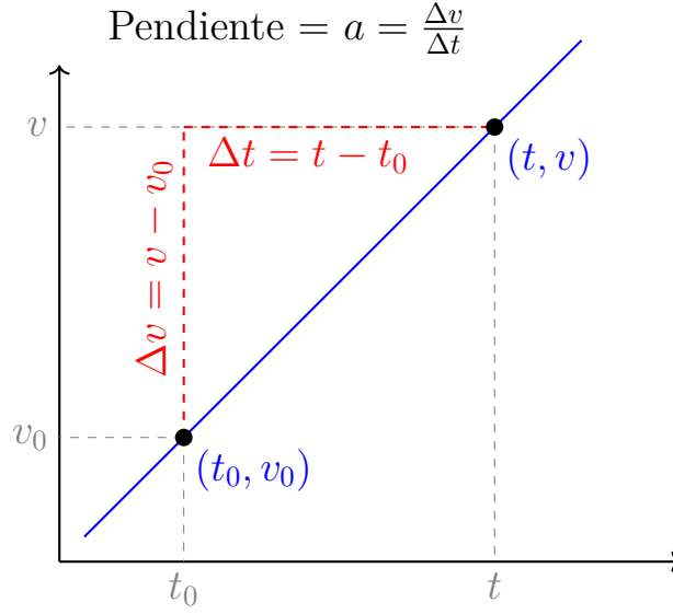
Figura 3.2: La aceleración como la pendiente de una línea recta en el plano de velocidad en función del tiempo
