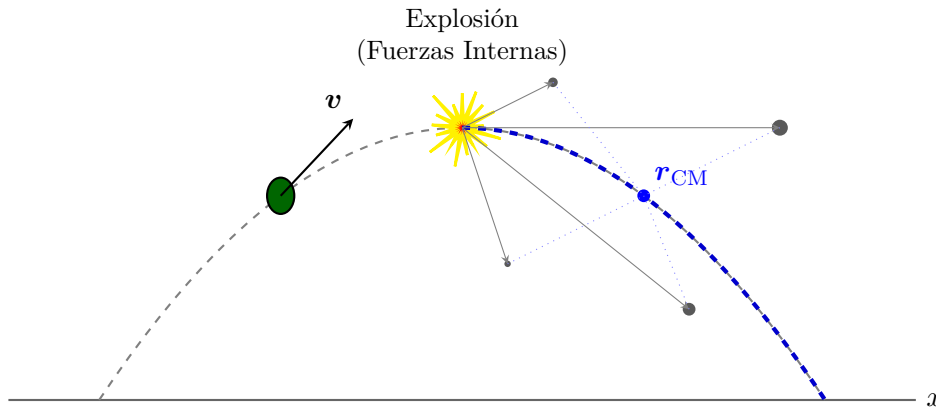
Figura 3.8: Explosión de un proyectil en movimiento parabólico. Aunque los fragmentos individuales (puntos grises) salen disparados en trayectorias complejas, el Centro de Masas del sistema (punto azul) continúa describiendo exactamente la misma parábola original.
