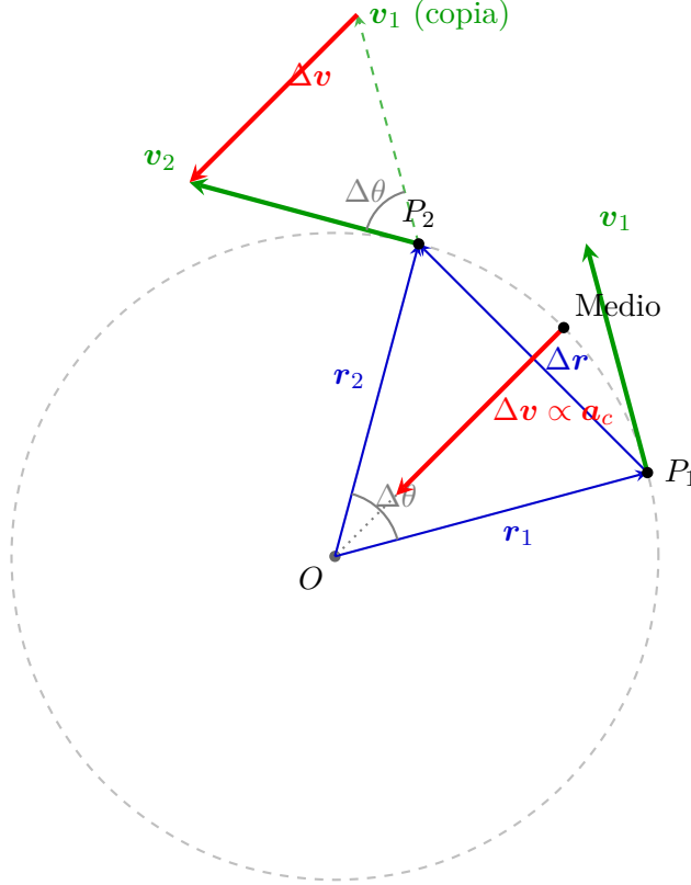
Figura 3.11: Derivación geométrica de la aceleración centrípeta en un único círculo. Al trasladar el vector \mathbf{v}_1 hacia P_2 , se forma el triángulo de velocidades que define \Delta\mathbf{v} . Si duplicamos este vector \Delta\mathbf{v} y lo ubicamos en el punto medio del desplazamiento espacial, observamos visualmente que se alinea a la perfección con la línea radial punteada, apuntando exactamente hacia el centro del círculo ( O ). Esto demuestra de forma irrefutable la naturaleza “centrípeta” (que busca el centro) de la aceleración.
