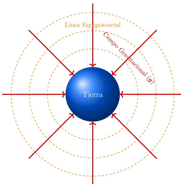
Figura 3.3: Representación en 2D del campo gravitacional ( \mathbf{g} ) generado por la Tierra. Las líneas de campo (flechas rojas) son radiales y apuntan hacia el centro de masa. Las líneas equipotenciales (círculos naranjas a trazos) son perpendiculares a las líneas de campo y representan regiones de igual potencial gravitacional.
