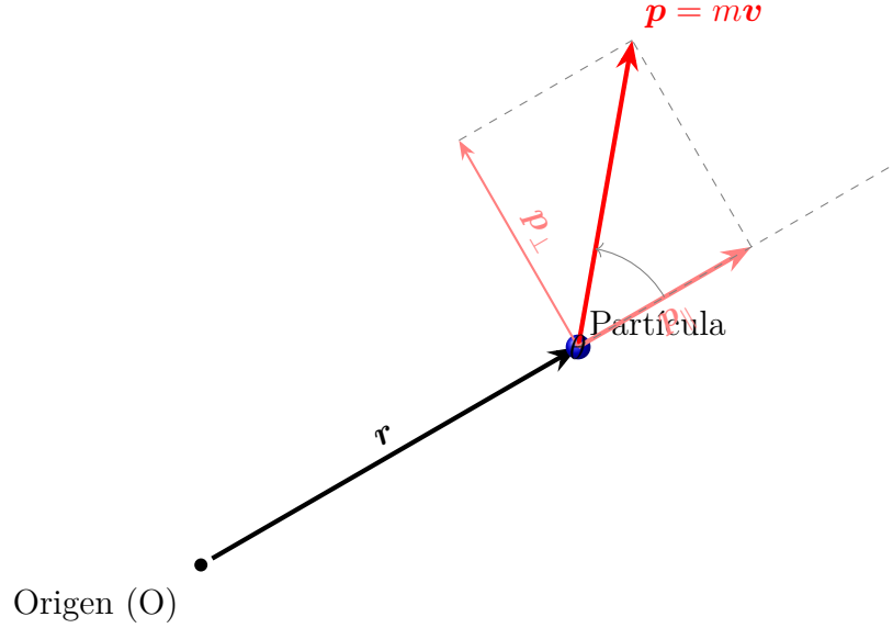
Figura 3.17: Ilustración mejorada de la definición de momento angular. El momento lineal \mathbf{p} se descompone en una componente paralela a \mathbf{r} ( \mathbf{p}_{\parallel} ) y una perpendicular ( \mathbf{p}_{\perp} ), ambas originadas en la partícula. El momento angular solo depende de la componente perpendicular: \mathbf{L} = \mathbf{r} \times \mathbf{p}_{\perp} . Su magnitud es L = |\mathbf{r}||\mathbf{p}_{\perp}| = r(p \sin \theta) .
