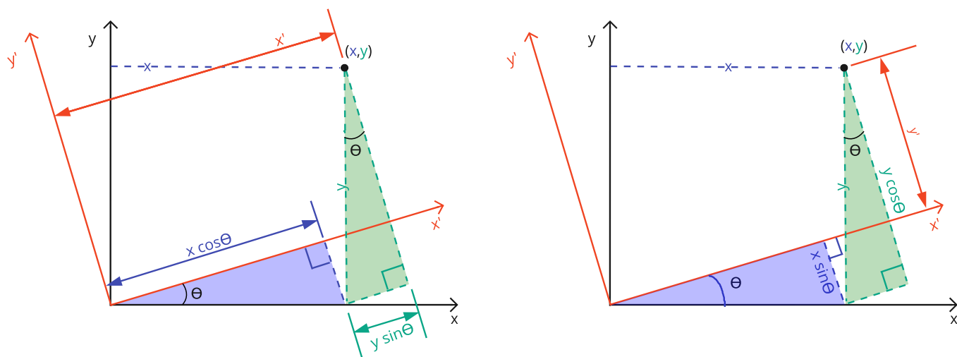
Figura 1.1: Rotación de sistema de coordenadas
