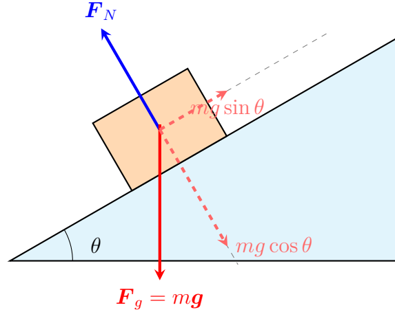
Figura 3.11: Diagrama de cuerpo libre para un bloque en un plano inclinado moviéndose hacia abajo. La fuerza gravitacional ( F_g ) se descompone en una componente perpendicular ( mg \cos \theta ) y una componente paralela ( mg \sin \theta ) al plano.
