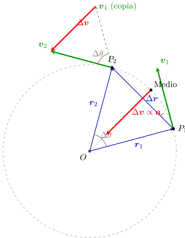
Figura 3.13: Derivación geométrica de la aceleración centrípeta en un único círculo. Al trasladar el vector v_1 hacia P_2 , se forma el triángulo de velocidades que define \Delta v . Si duplicamos este vector \Delta v y lo ubicamos en el punto medio del desplazamiento espacial, observamos visualmente que se alinea a la perfección con la línea radial punteada, apuntando exactamente hacia el centro del círculo ( O ). Esto demuestra de forma irrefutable la naturaleza “centrípeta” (que busca el centro) de la aceleración.
