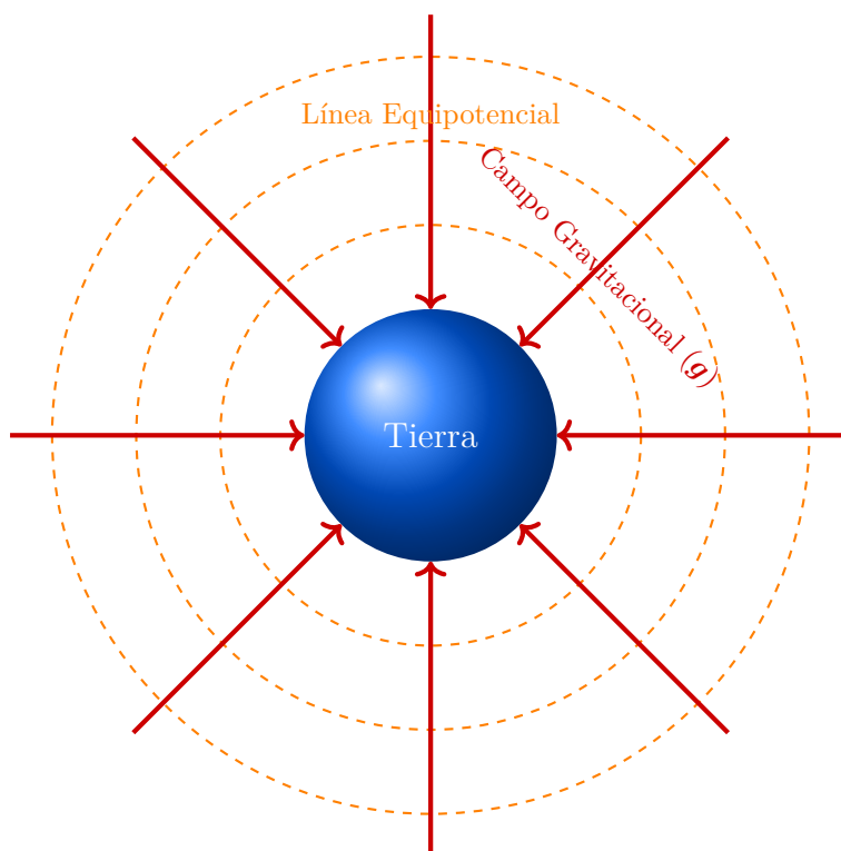
Figura 3.5: Representación en 2D del campo gravitacional ( g ) generado por la Tierra. Las líneas de campo (flechas rojas) son radiales y apuntan hacia el centro de masa. Las líneas equipotenciales (círculos naranjas a trazos) son perpendiculares a las líneas de campo y representan regiones de igual potencial gravitacional.
