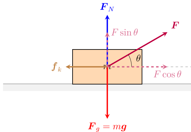
Figura 3.12: Diagrama de cuerpo libre para un bloque sobre una superficie horizontal con fricción, sujeto a una fuerza \mathbf{F} aplicada con un ángulo \theta . Se muestran todas las fuerzas y la descomposición de la fuerza aplicada.
