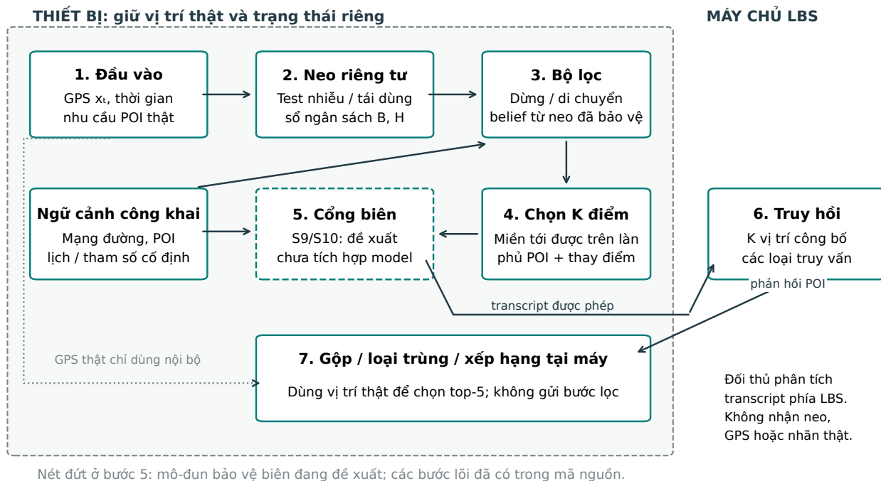
Hình 2. Kiến trúc lỗi đã có trong mã nguồn và vị trí dự kiến của cổng bảo vệ biên S9/S10. Neo và nhãn thật không thuộc transcript máy chủ.
