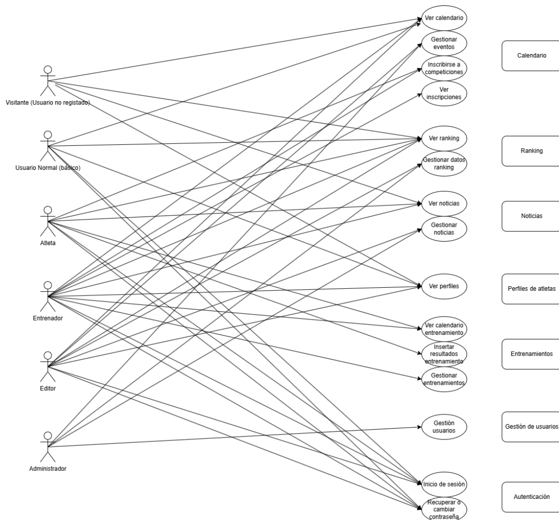
[Fig 4: Diagrama de casos de uso de la aplicación]
