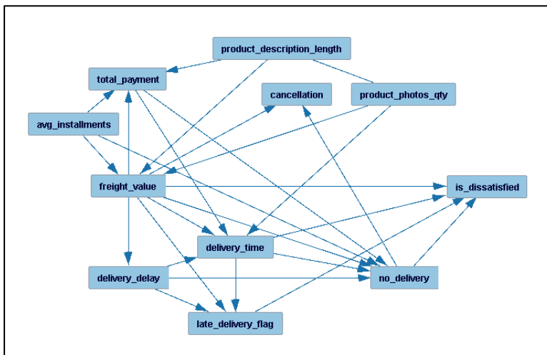
m. DAG cluster 1
