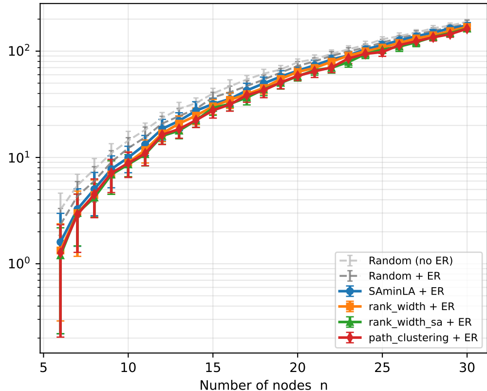
CNOTs
