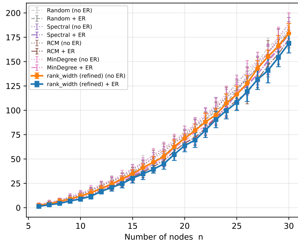
CNOTs
