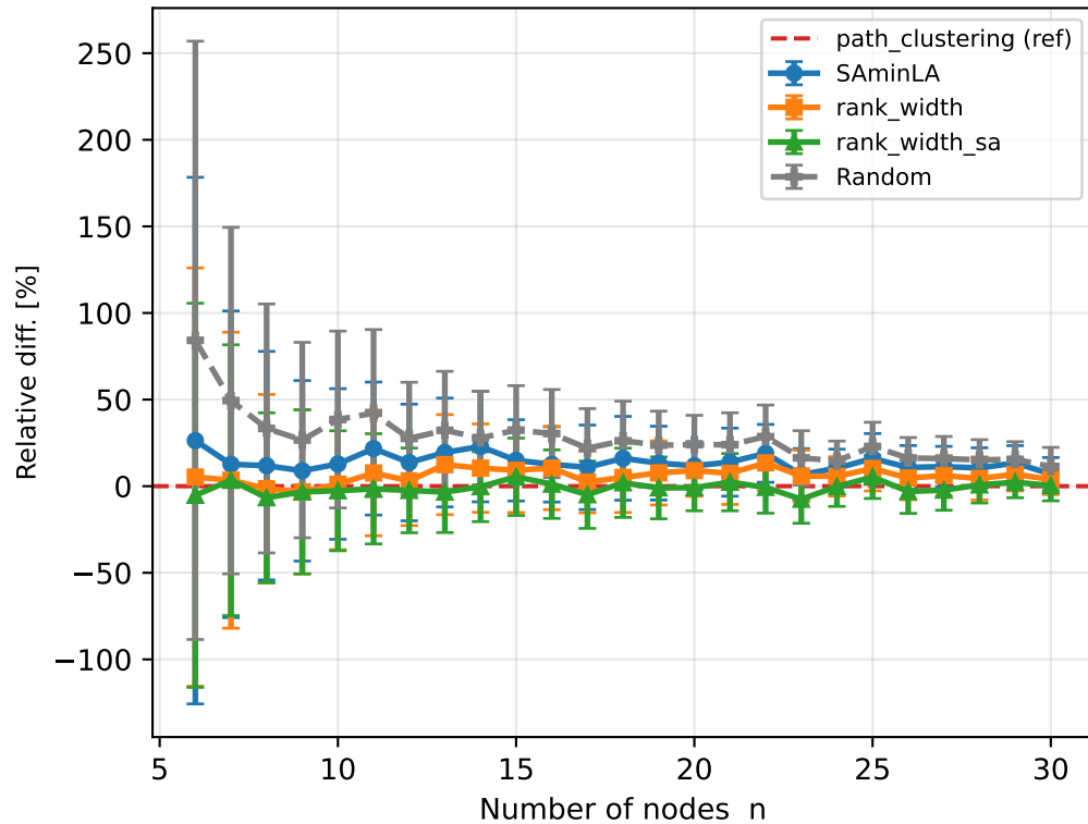
CNOTs
