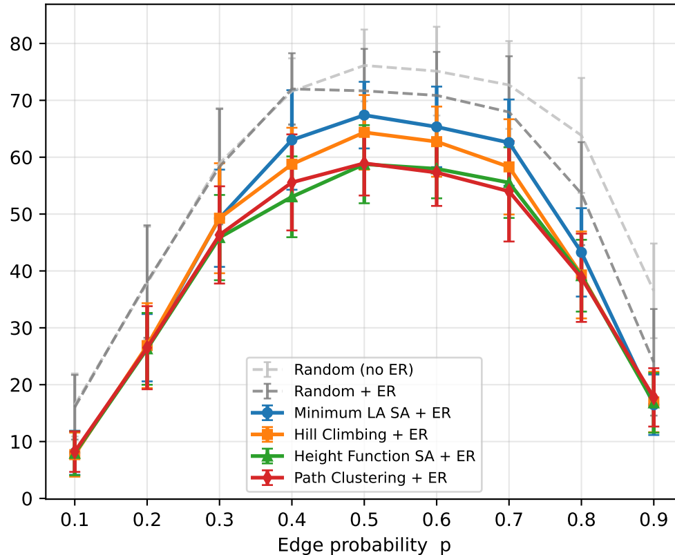
CNOTs
