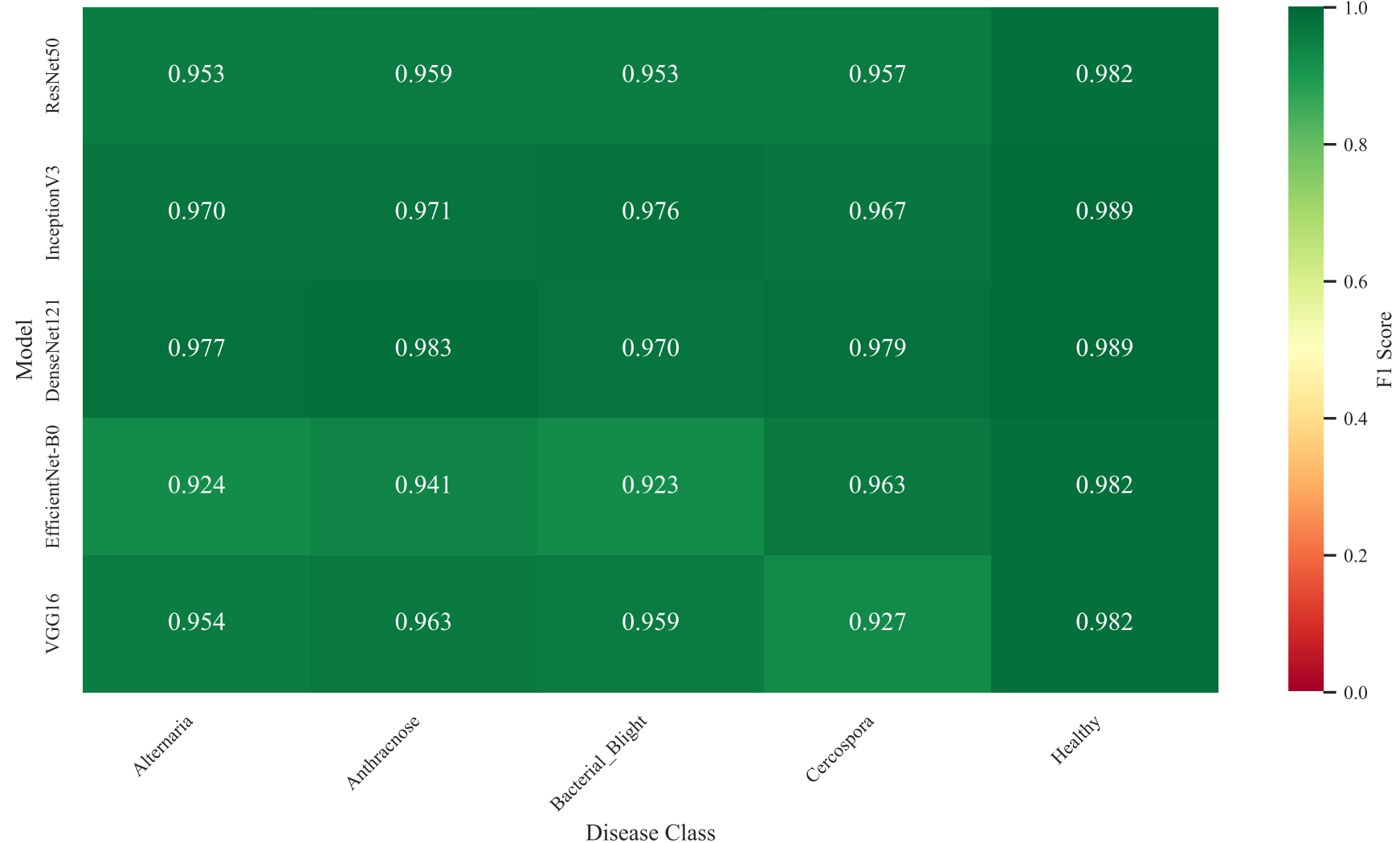
Per-Class F1 Scores (Test Set)
