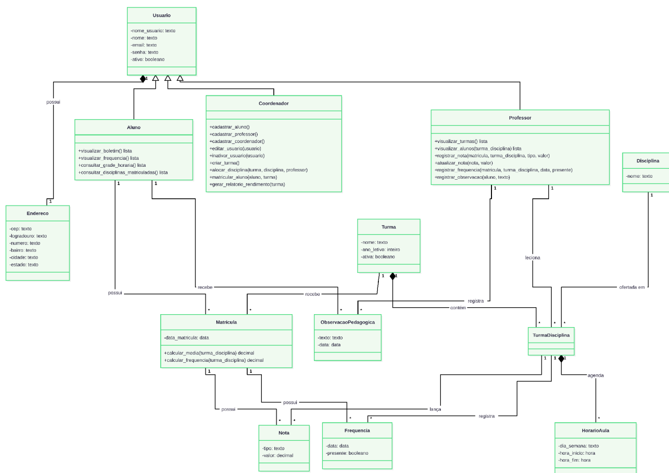
Figura 1 — Diagrama de classes (UML) do Sistema de Gestão Escolar.
