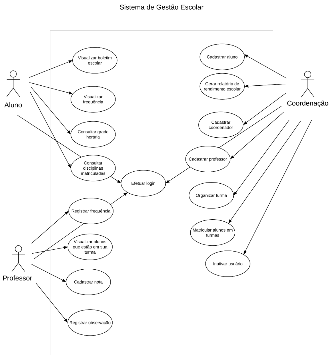
Figura 1 : Diagrama de casos de uso (UML) do Sistema de Gestão Escolar.
