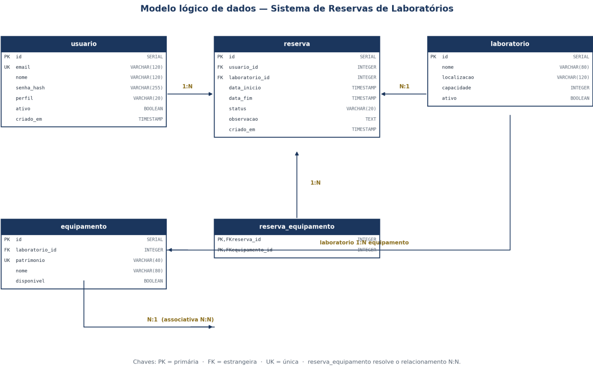
Figura 1 — Modelo lógico (tabelas e integridade referencial).
