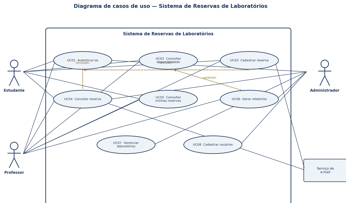
Figura 1 — Diagrama de casos de uso (UML) do exemplo acadêmico.
