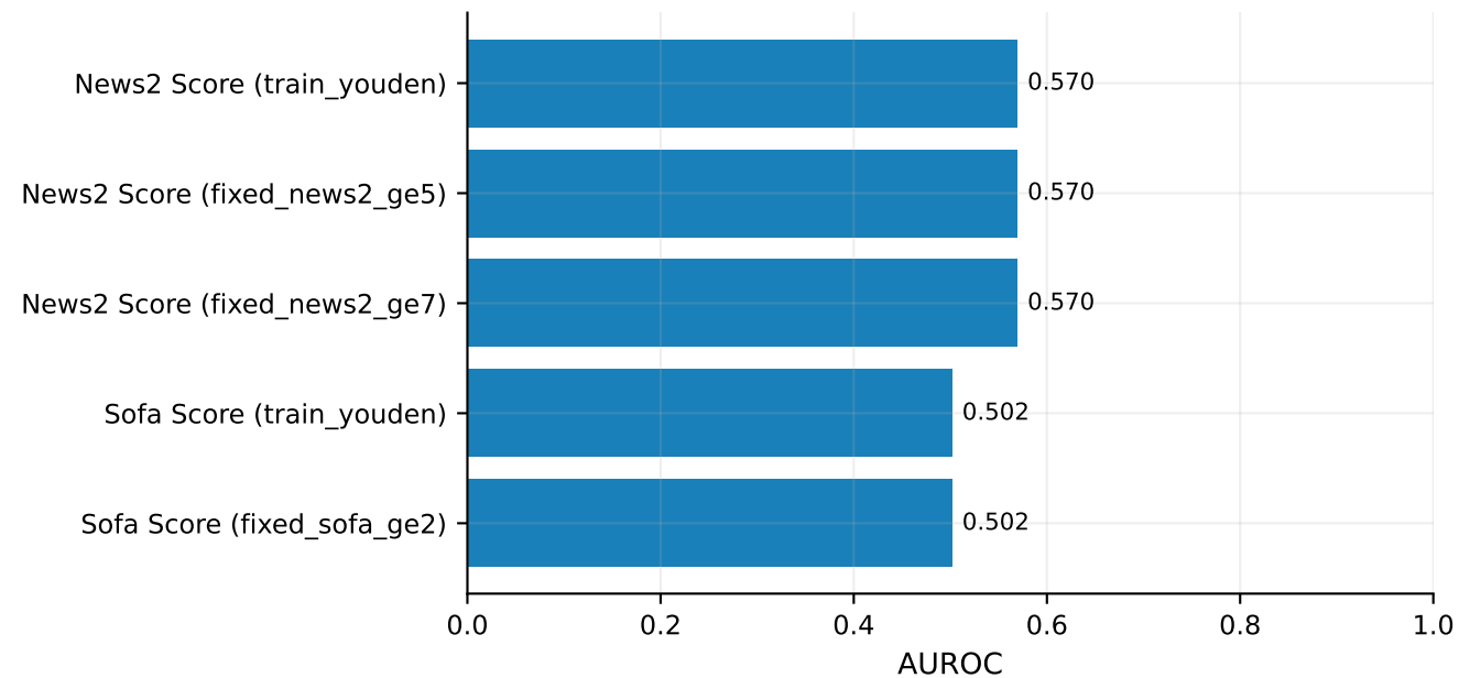
AUROC
