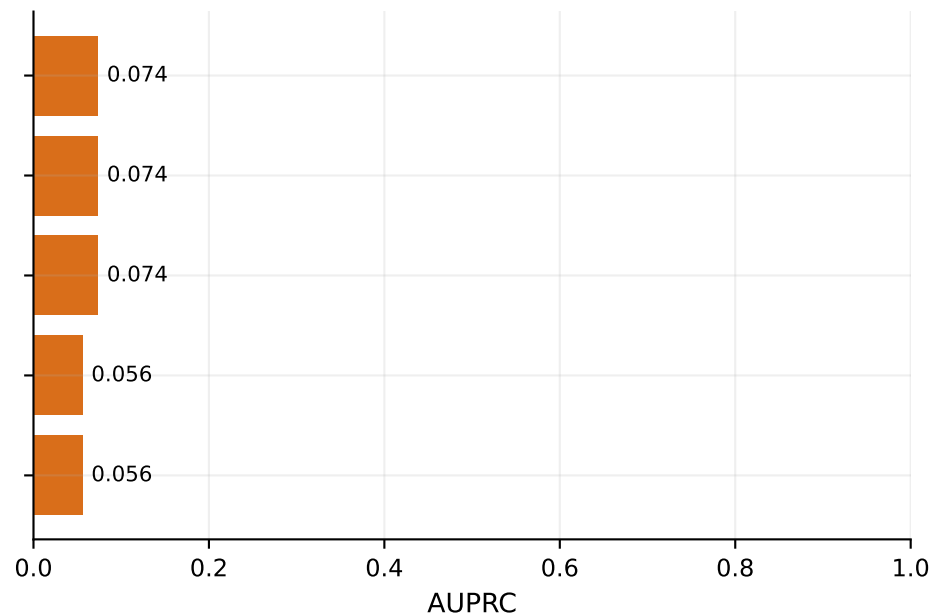
AUPRC
