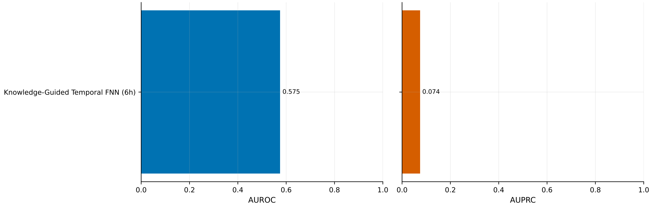
AUROC
