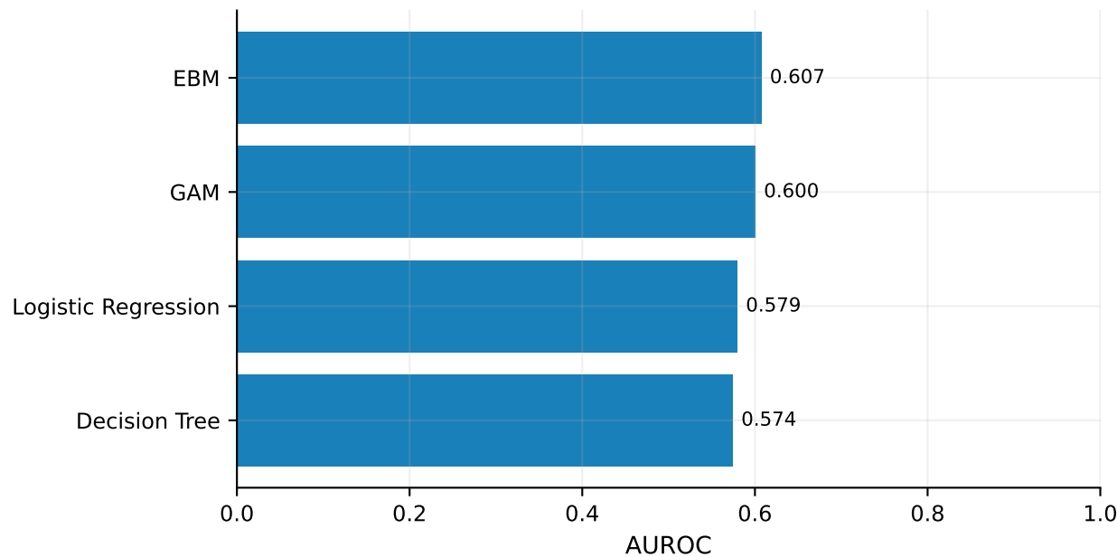
AUROC
