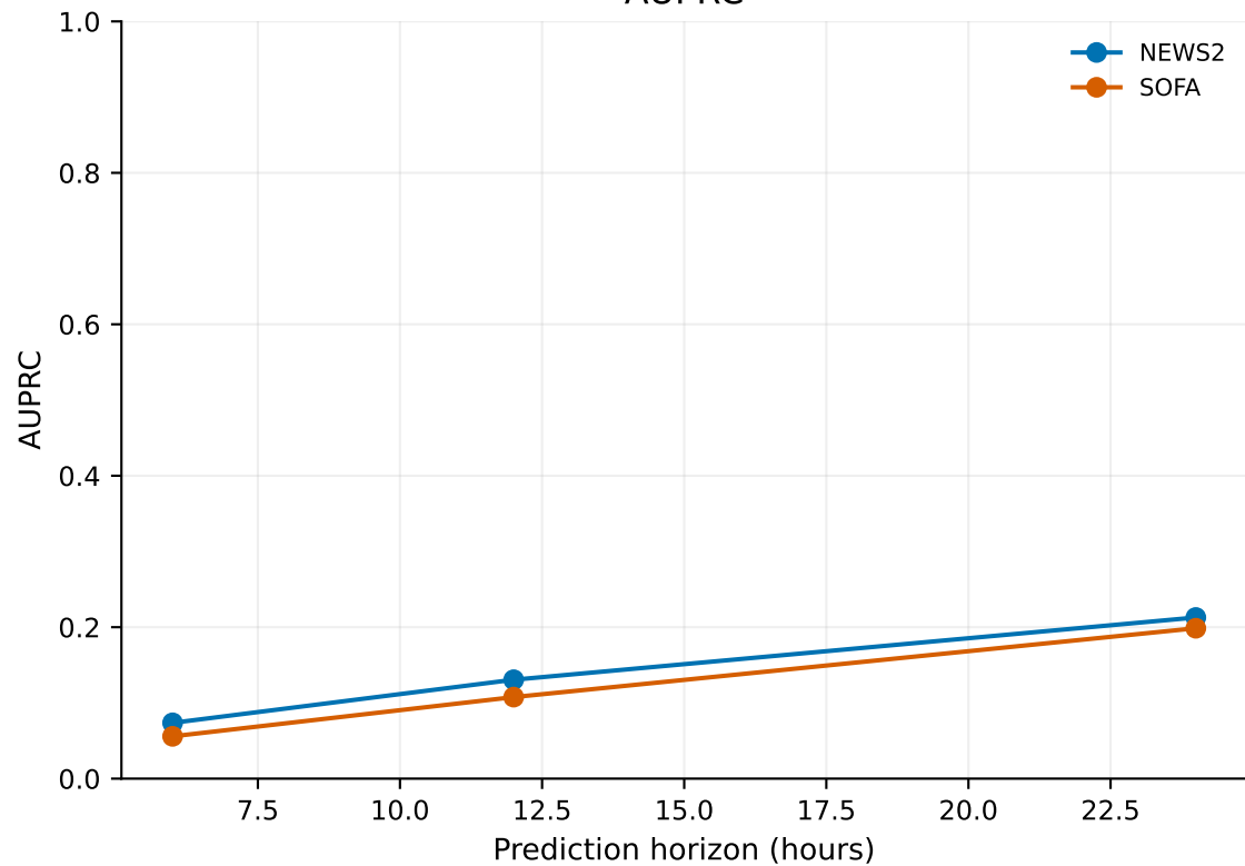
AUPRC
