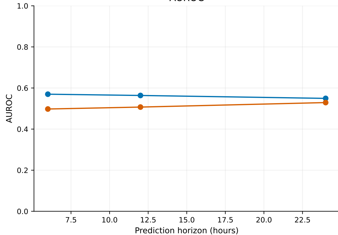
AUROC
