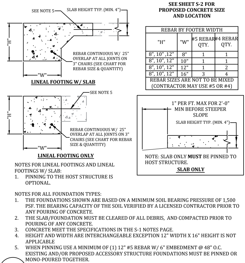
FOUNDATION DETAIL SCALE: N.T.S.
